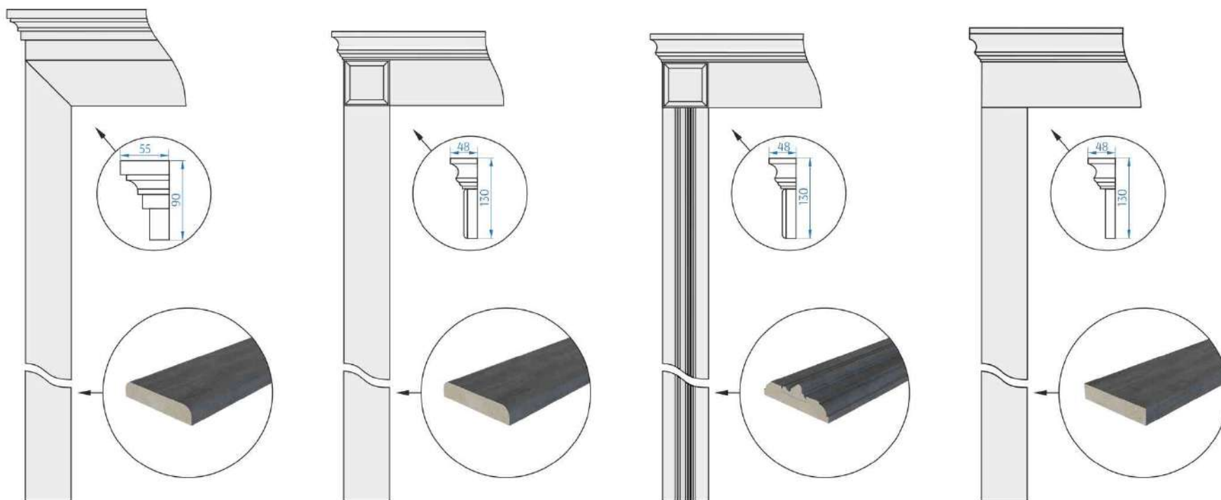
Карнизный модуль 01, наличник 01
